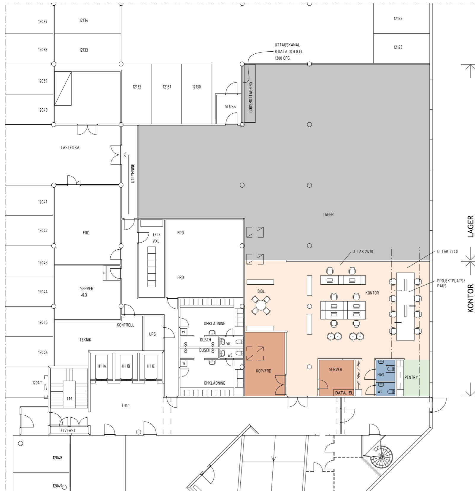
PLAN VÅNING 2
