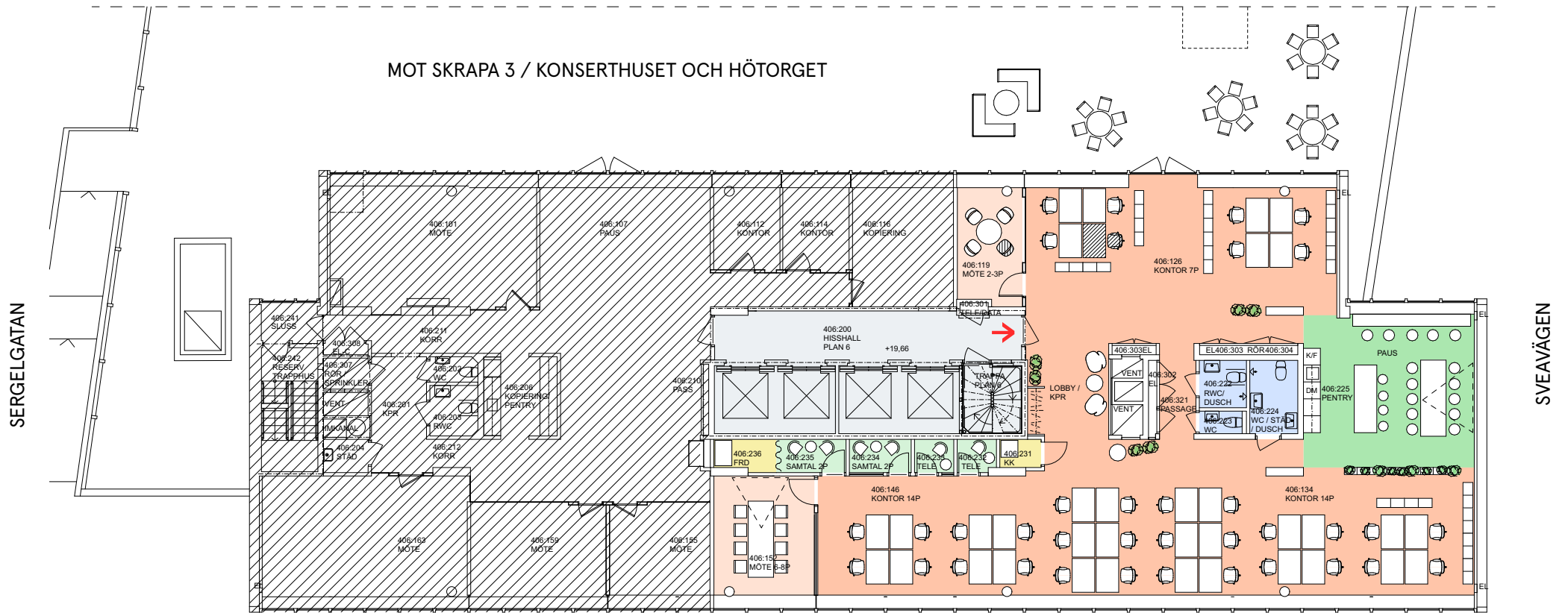
PLAN 6, VÅN. 2 TR.
